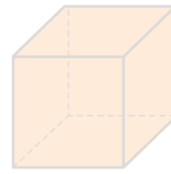
un cube
