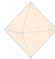
un octaèdre
