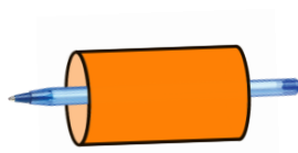
un cylindre
