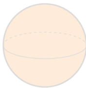
une sphère
